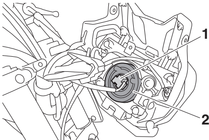
1. Fiche rapide de phare 2. Protection de l'ampoule de phare
